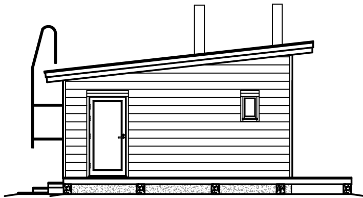
Julkisivu, koillinen
