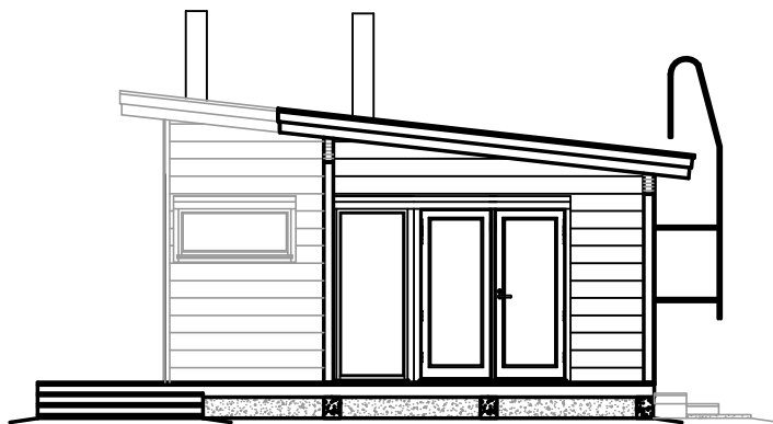
Julkisivu, lounas
