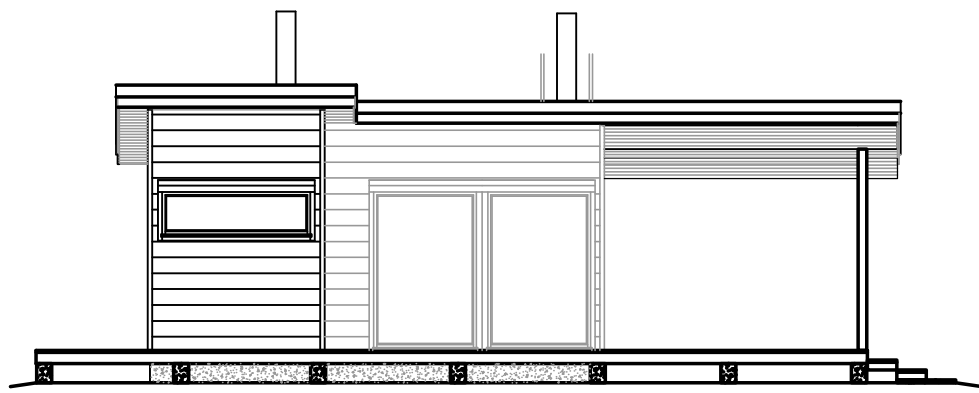
Julkisivu, luode
