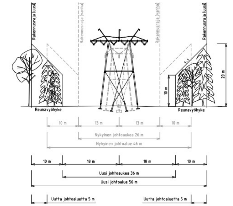
Kuva 2. Suunnitellun voimajohdon poikkileikkaus
