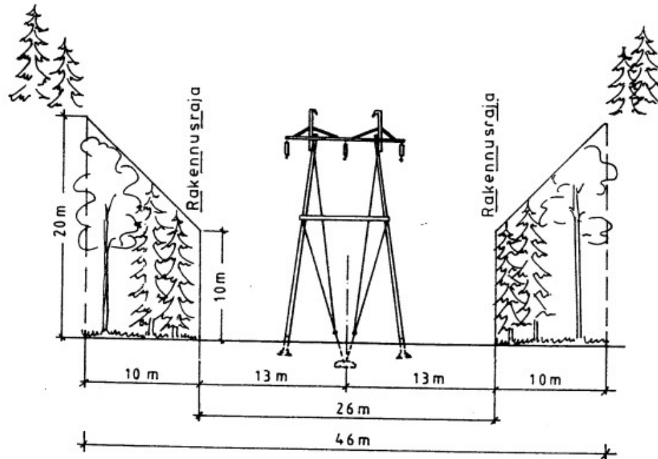
Kuva 1. Voimajohdon poikkileikkaus
