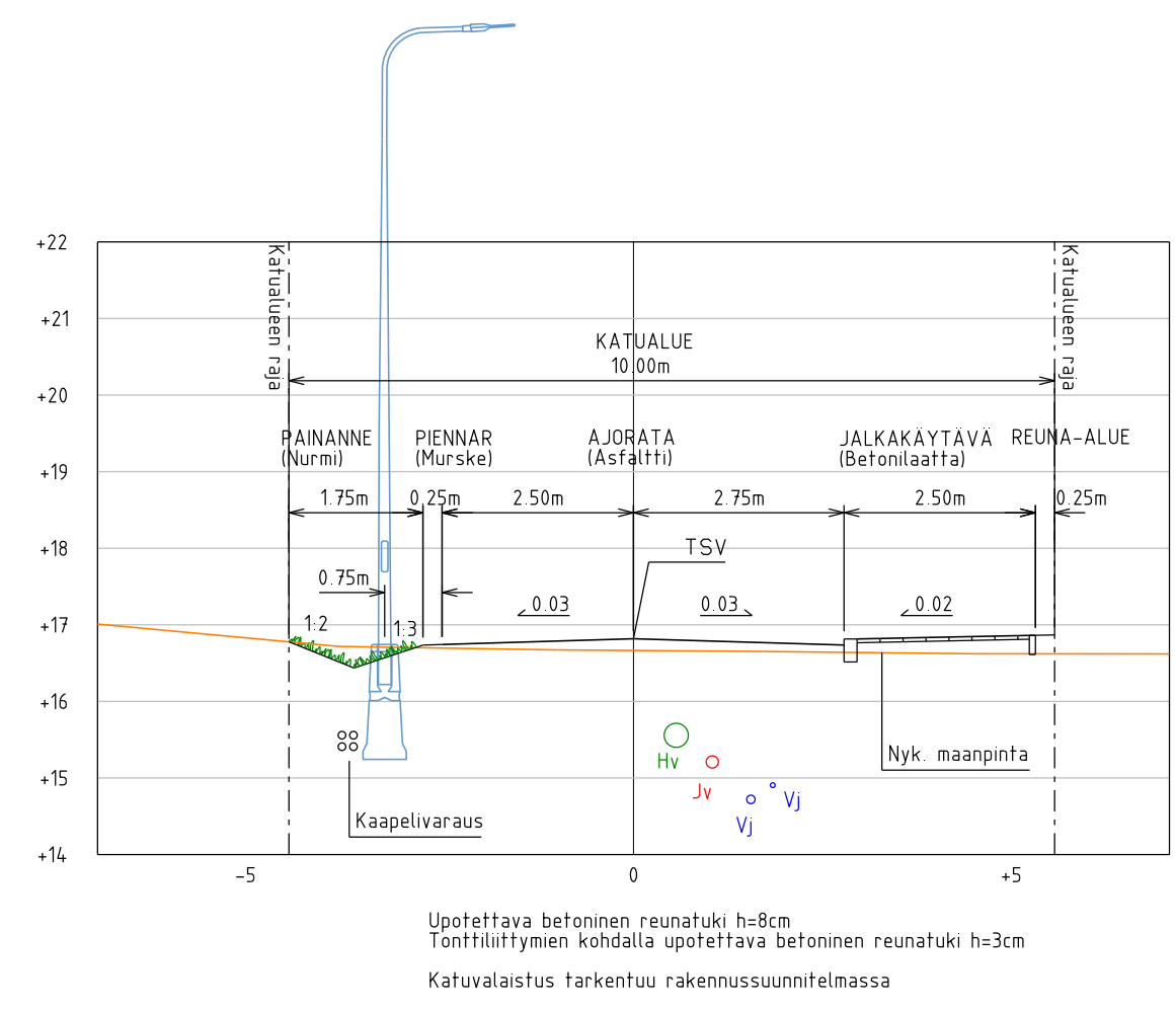
Tyyppipoikkileikkaus Ranta-ahde paalu 60 1:100/1:100
